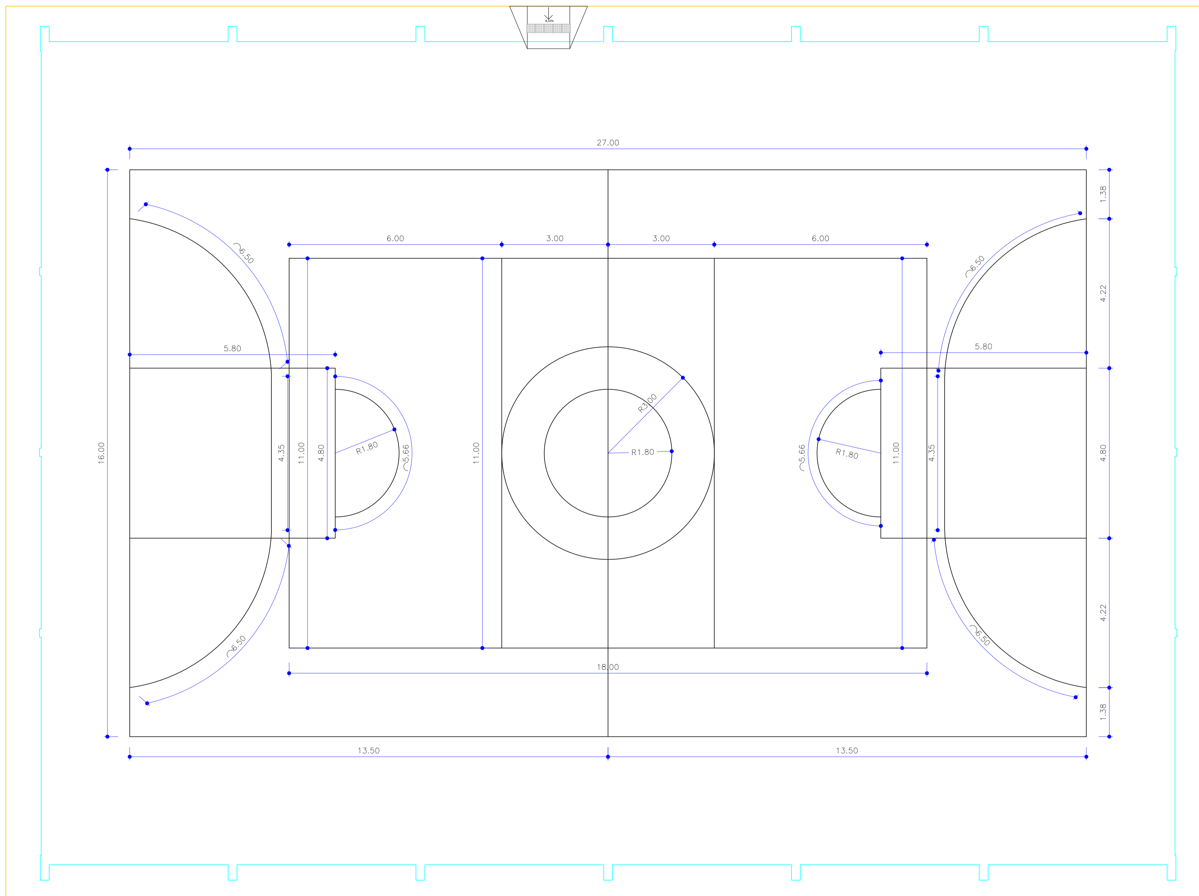
PLANTA DE PINTURA Esc: 1/65
