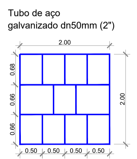
6 DETALHAMENTO PORTEIRA MOD. 02 ESC: 1/75
