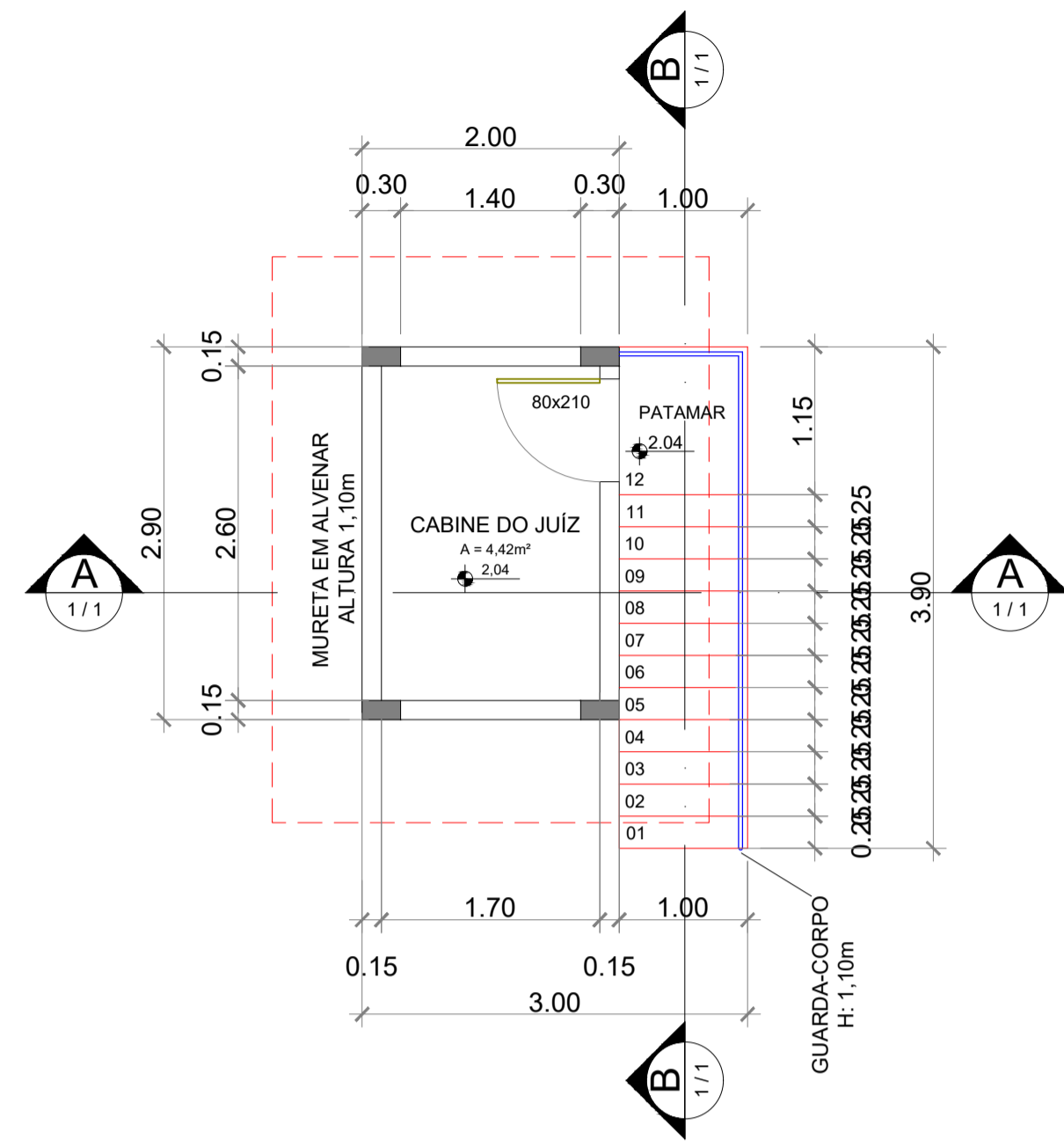
1 PLANTA BAIXA CABINE ESC: 1/50
