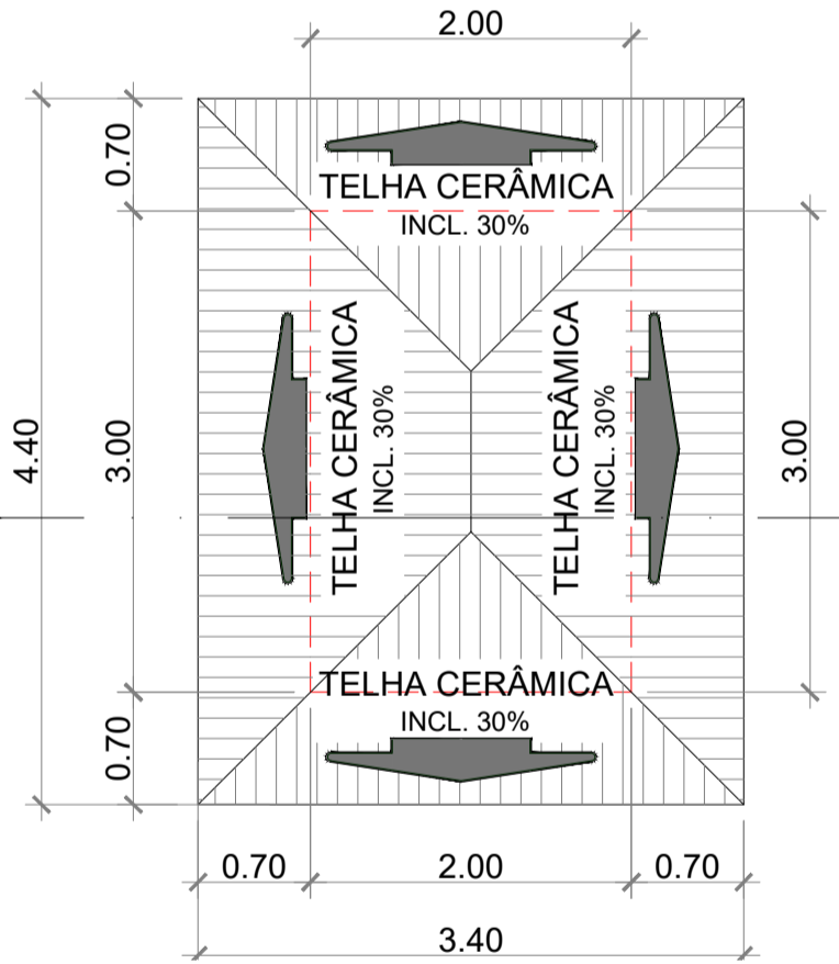
3 PLANTA DE COBERTURA ESC: 1/50
