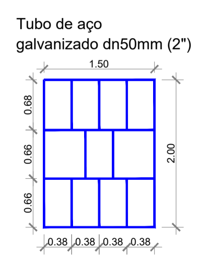
7 DETALHAMENTO PORTEIRA MOD. 01 ESC: 1/75
