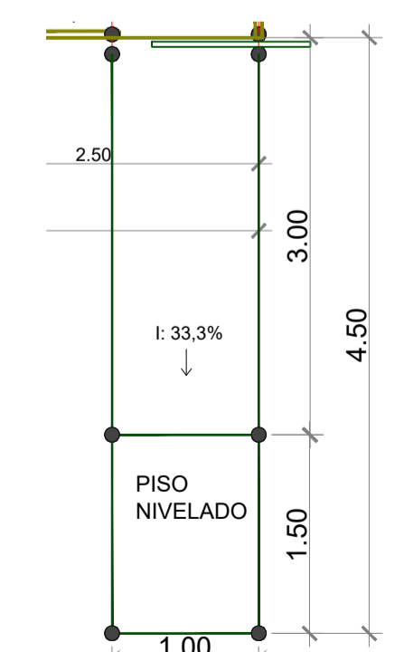
8 DETALHAMENTO EMBARCADOR DE GADO ESC: 1/50
