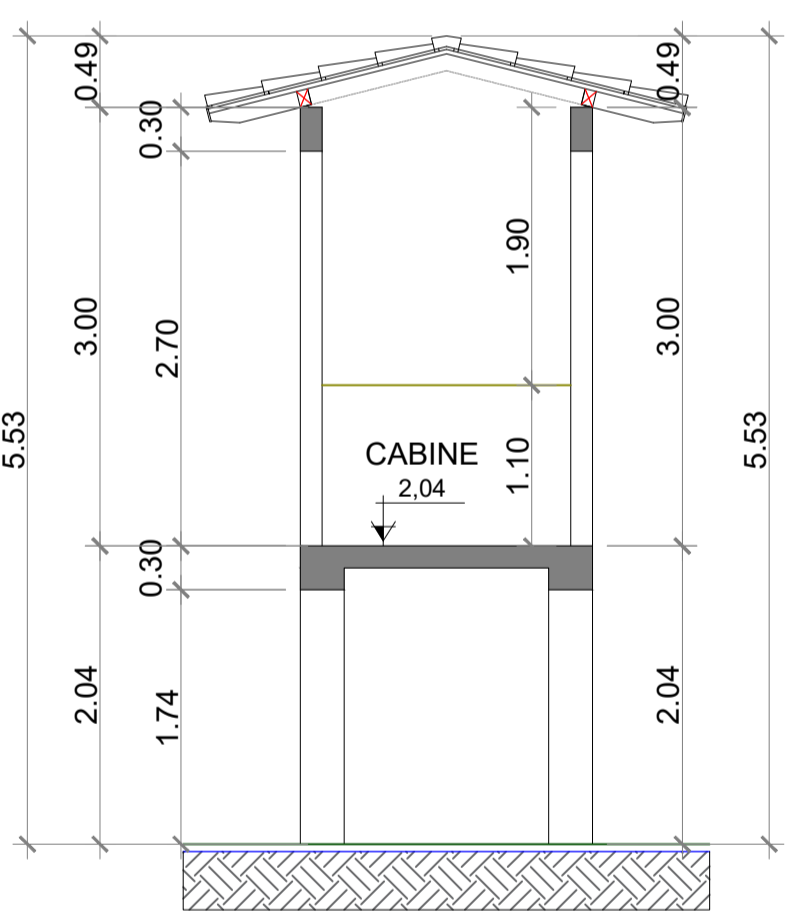
4 CORTE A-A ESC: 1/50
