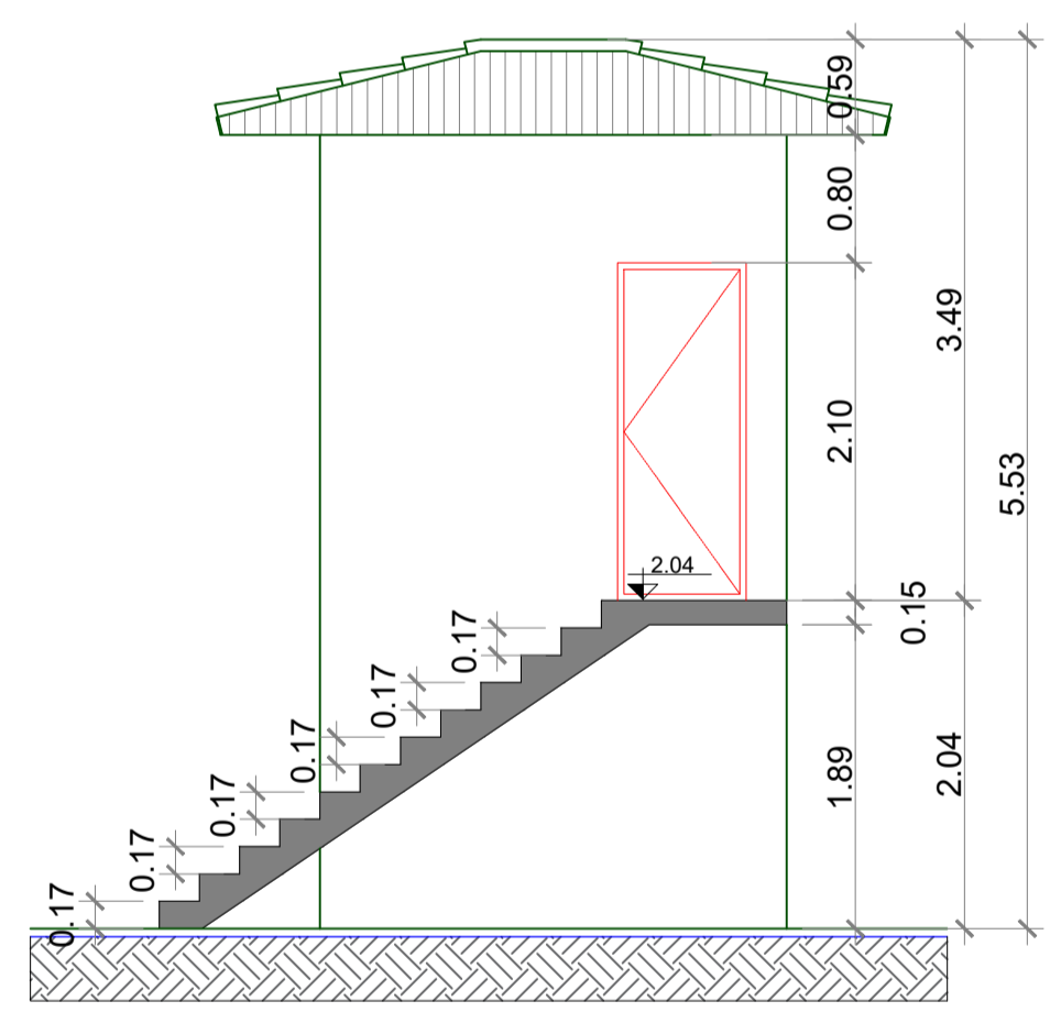
5 CORTE B-B ESC: 1/50
