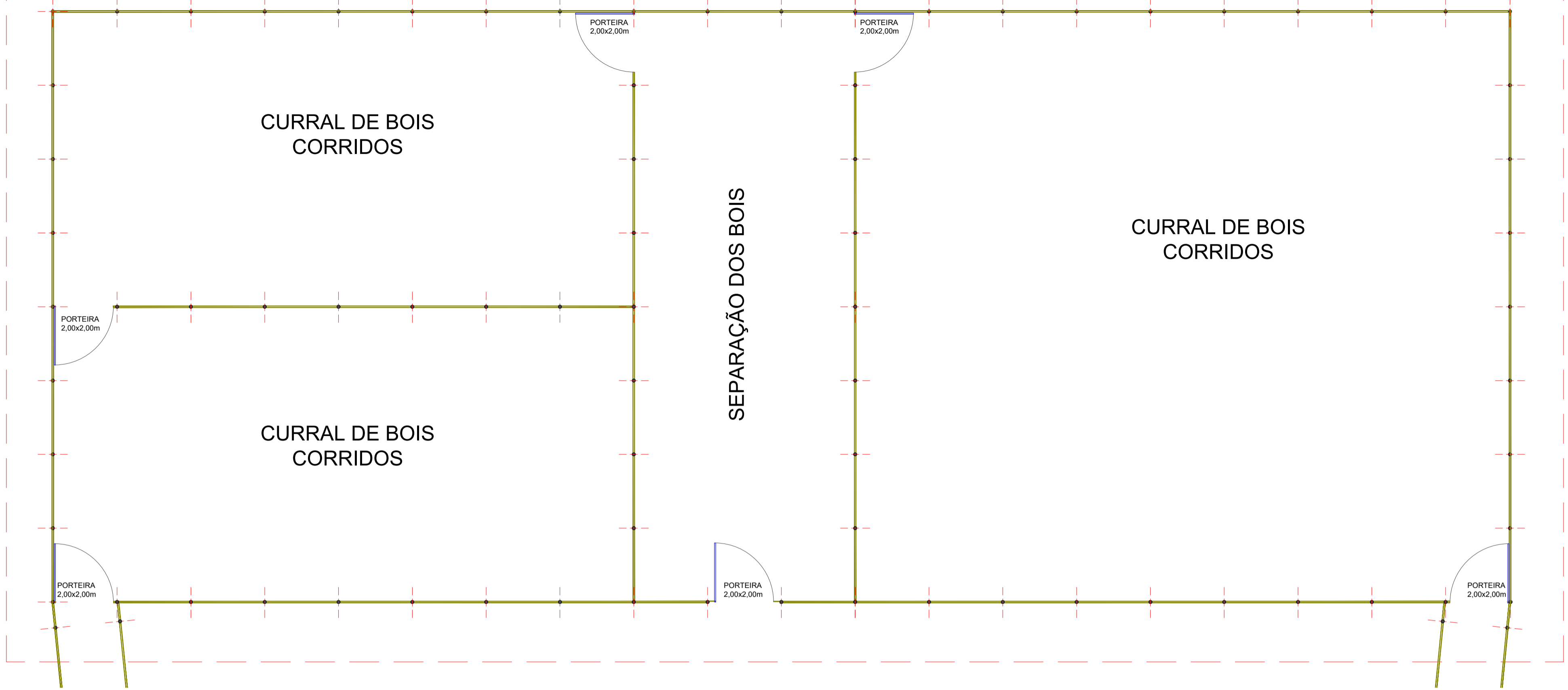
2 PLANTA BAIXA PISTA DE VAQUEIJADA - PARTE 02 ESC: 1/100
