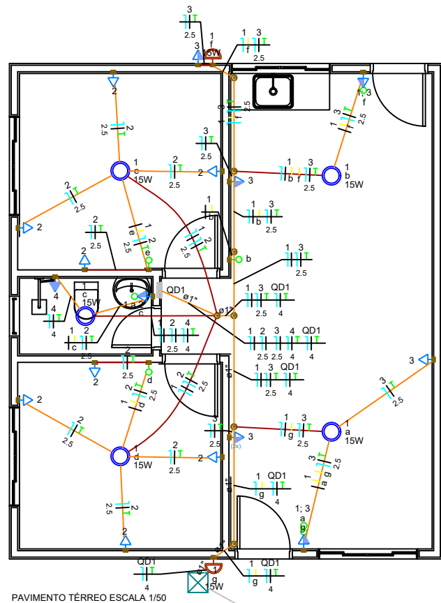
PAVIMENTO TÉRREO ESCALA 1/50
