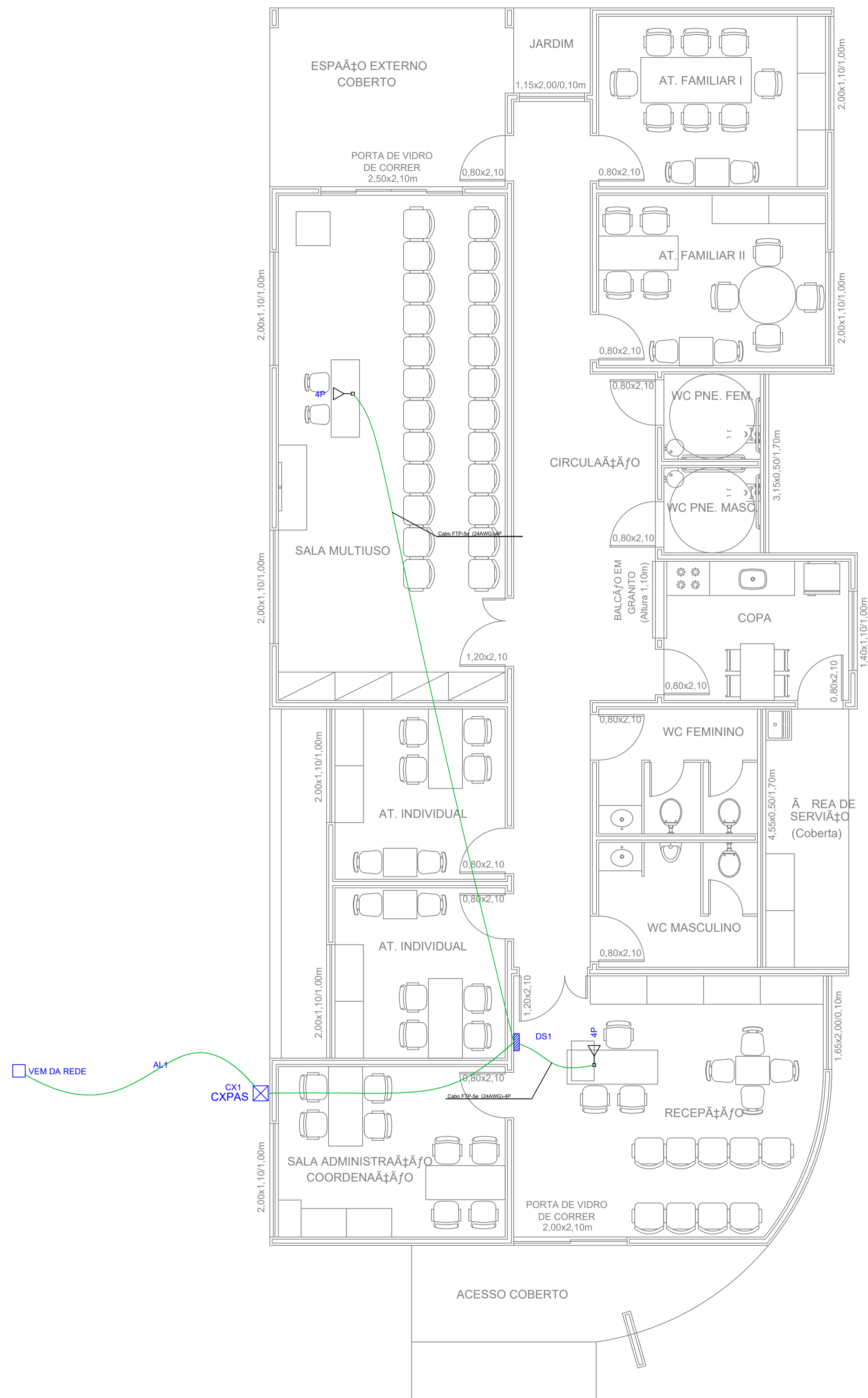
PLANTA BAIXA TELEFÔNICA ESCALA 1:50
