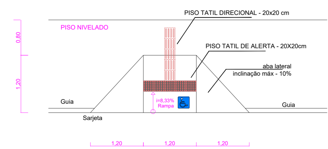
DETALHE DA RAMPA DE ACESSIBILIDADE ESC: 1/50
