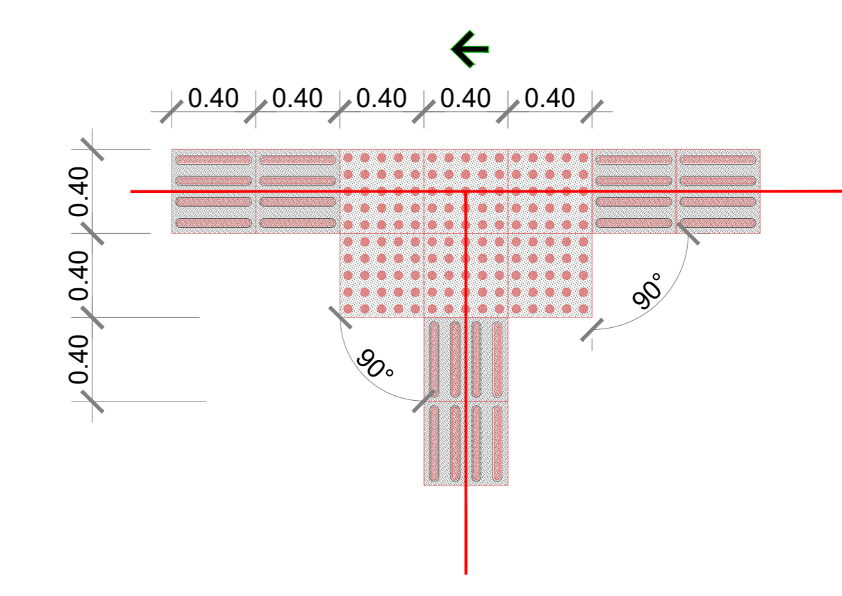
DETALHE PISO TÁTIL ESC: 1/50
