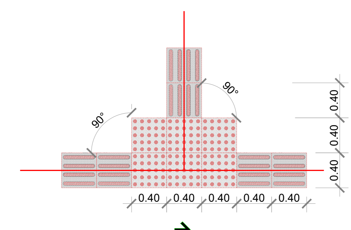
DETALHE PISO TÁTIL ESC: 1/50
