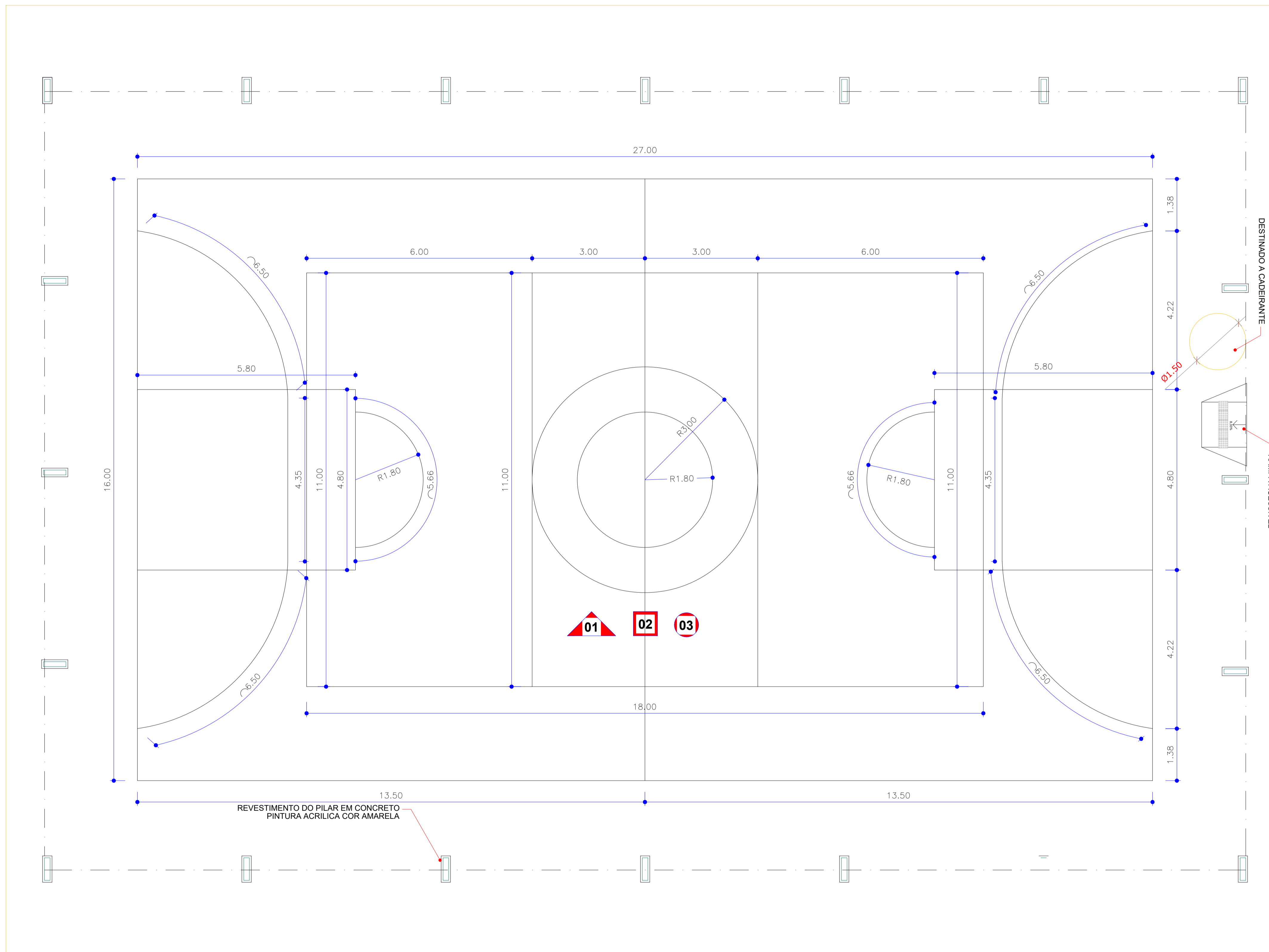
PLANTA DE PINTURA Esc: 1/60
