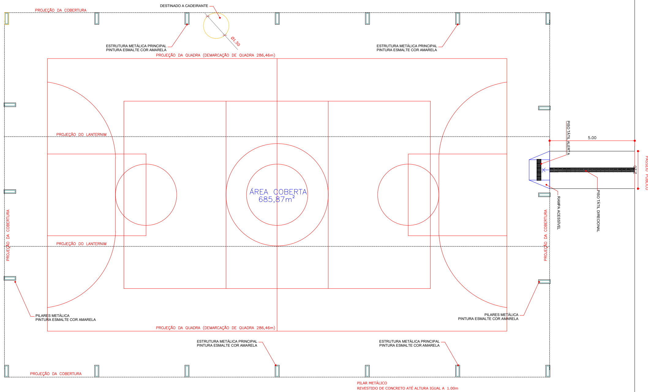
PLANTA BAIXA ESCALA 1:125
