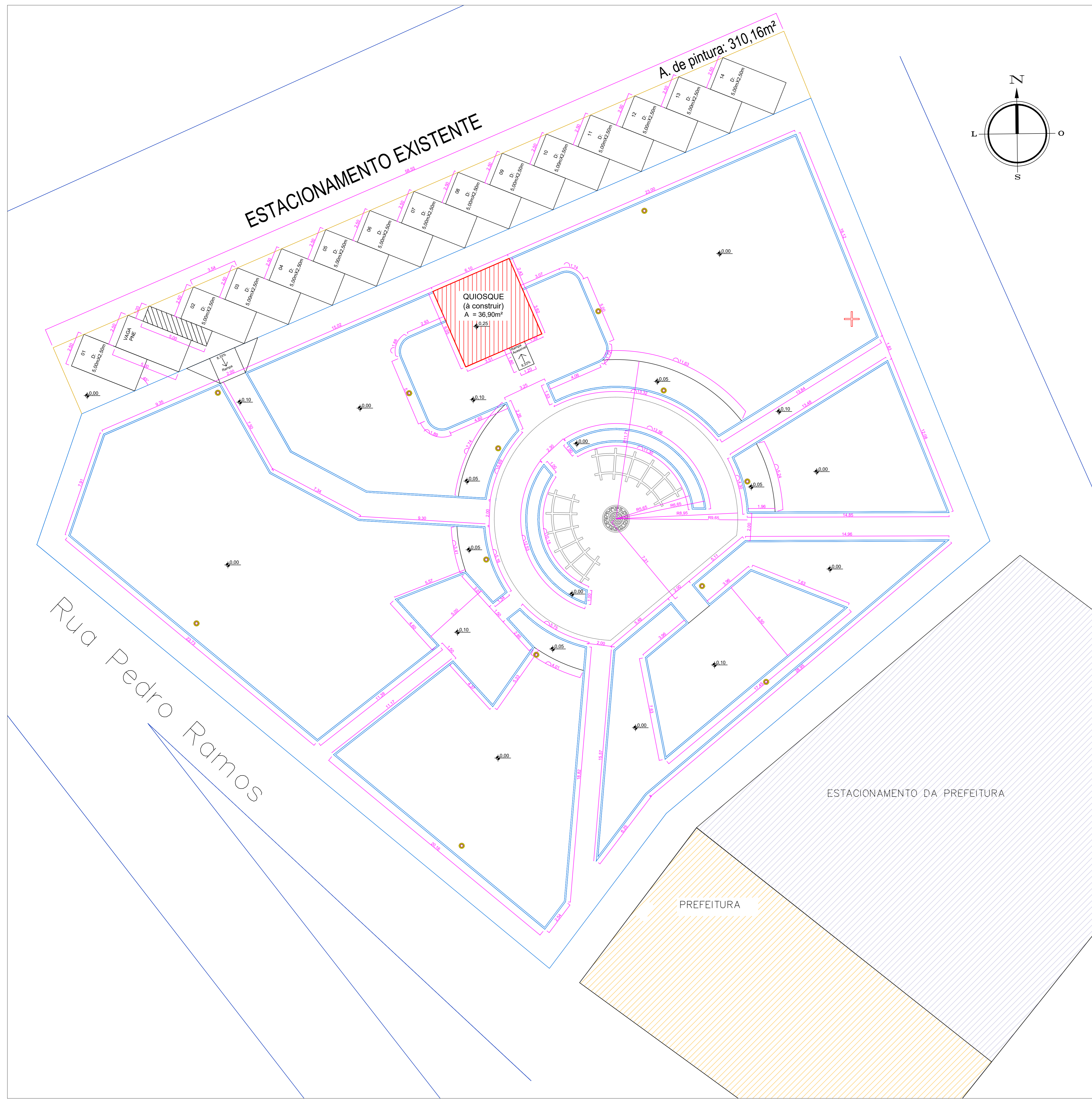
PLANTA DE LOCAÇÃO FINAL ESCALA: 1:150
