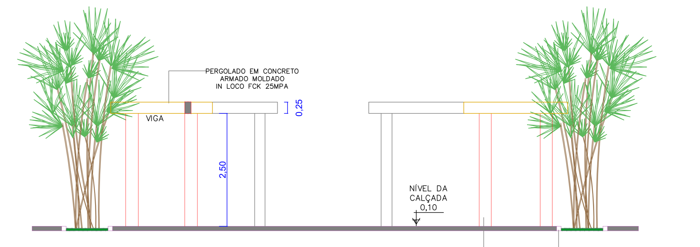
CORTE AA - PERGOLADO ESCALA: 1:50
