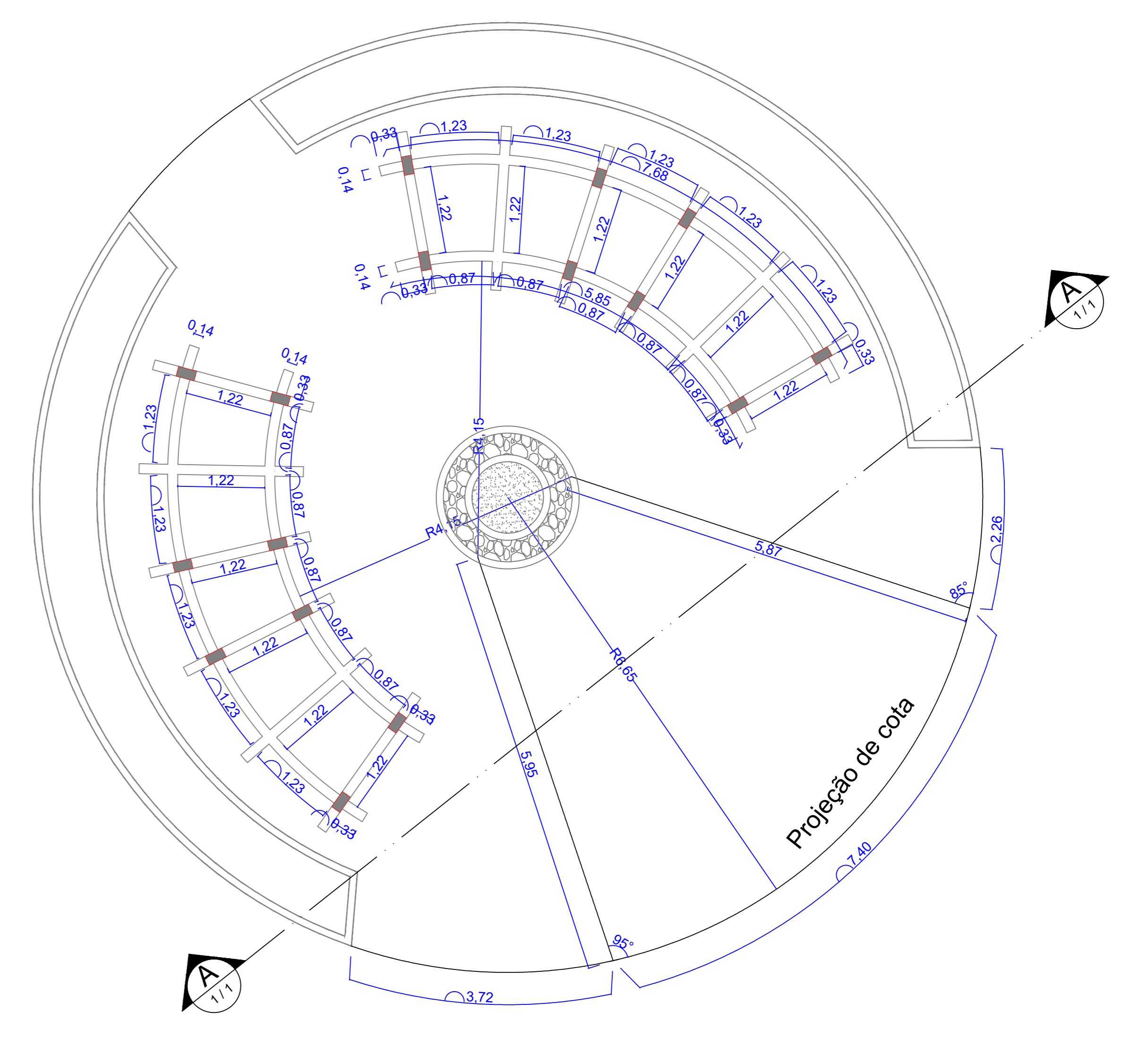
PLANTA BAIXA PERGOLADO ESCALA: 1:50
