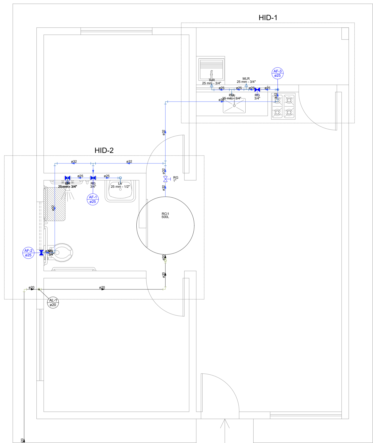
PLANTA BAIXA UNIDADE ISOLADA PCD ESCALA: 1:50
