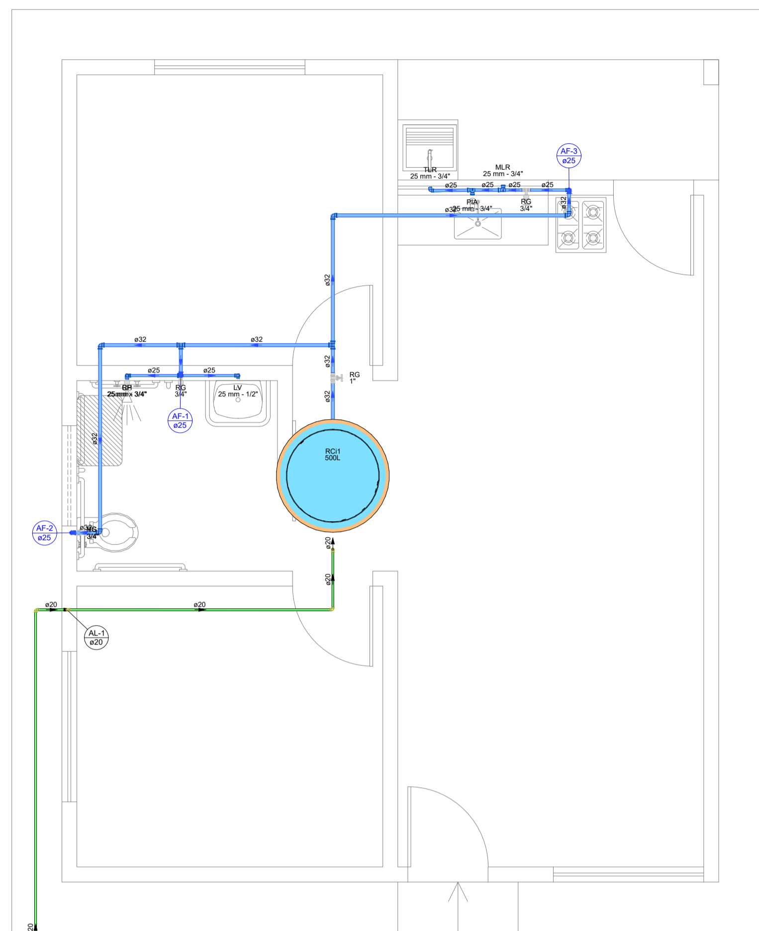
PLANTA BAIXA UNIDADE ISOLADA PCD ESCALA: 1:50
