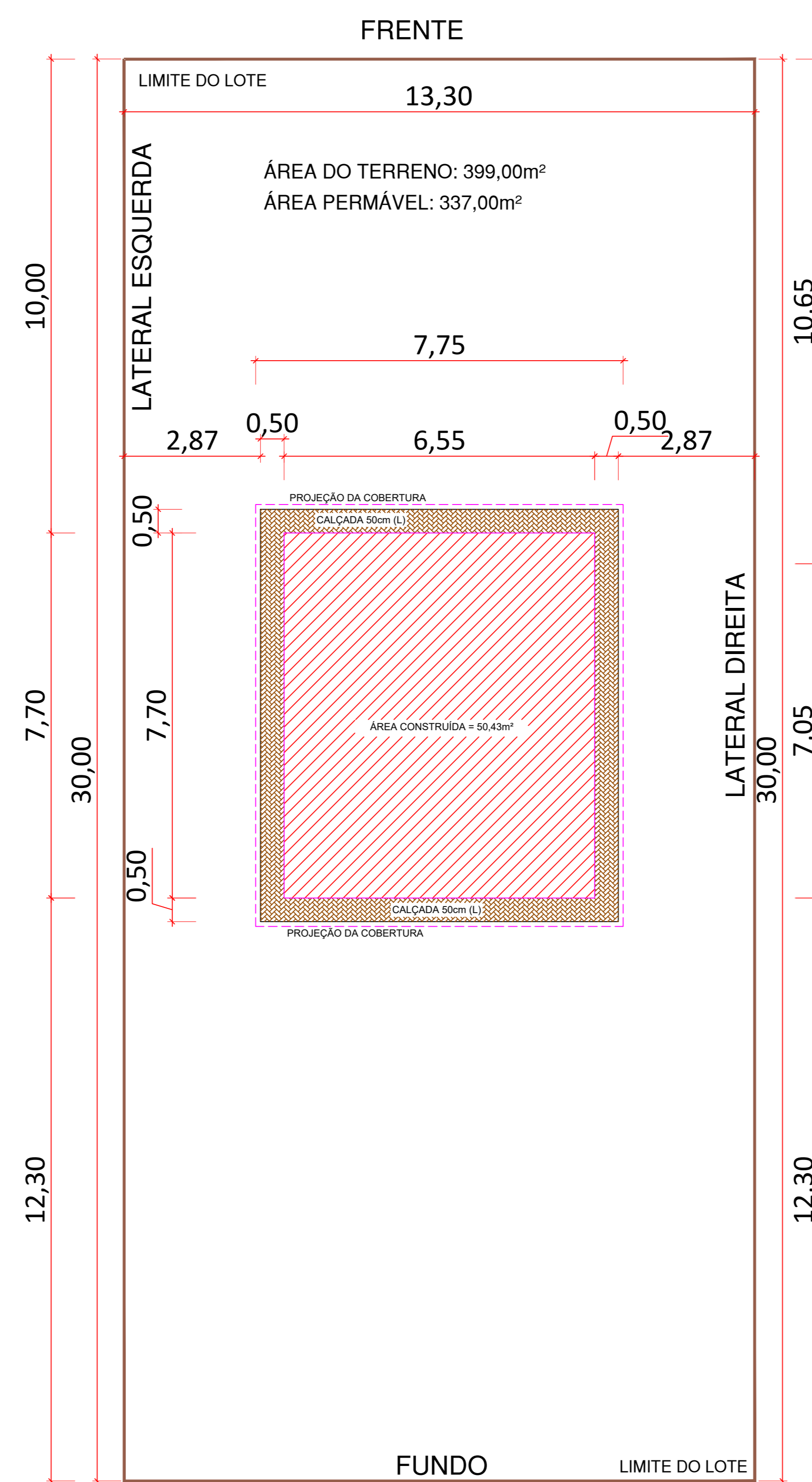
PLANTA DE LOCAÇÃO ESCALA: 1/75
