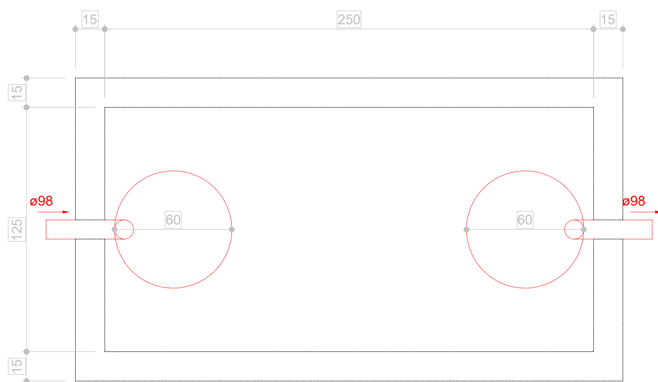
Tanque séptico - Cobertura Planta baixa - ESC. 1:25
