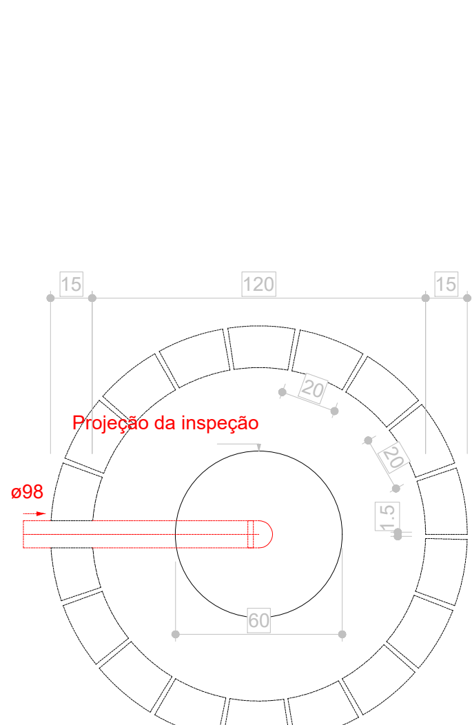
Sumidouro - Cobertura Planta baixa - ESC. 1:25
