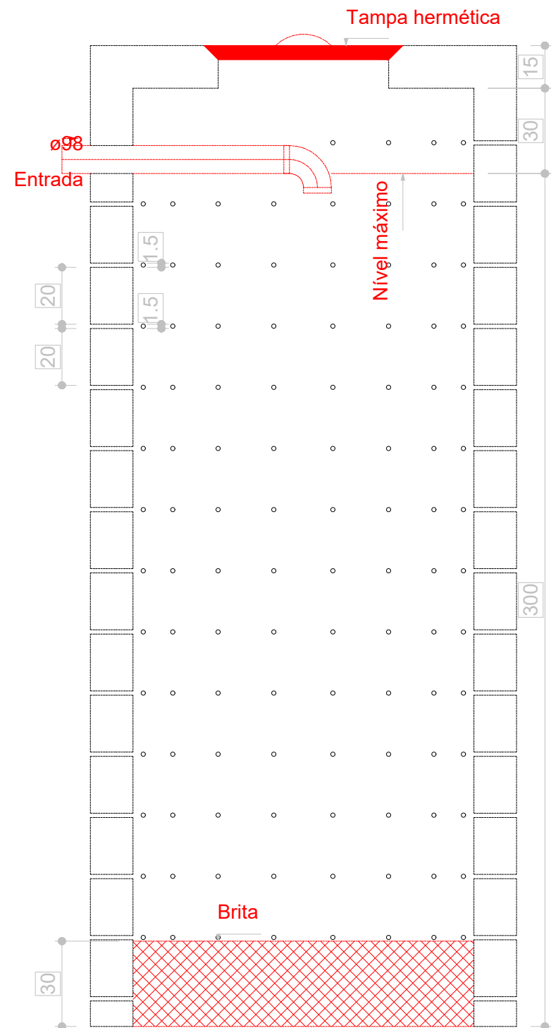
Sumidouro - Cobertura Corte 1 - ESC. 1:25
