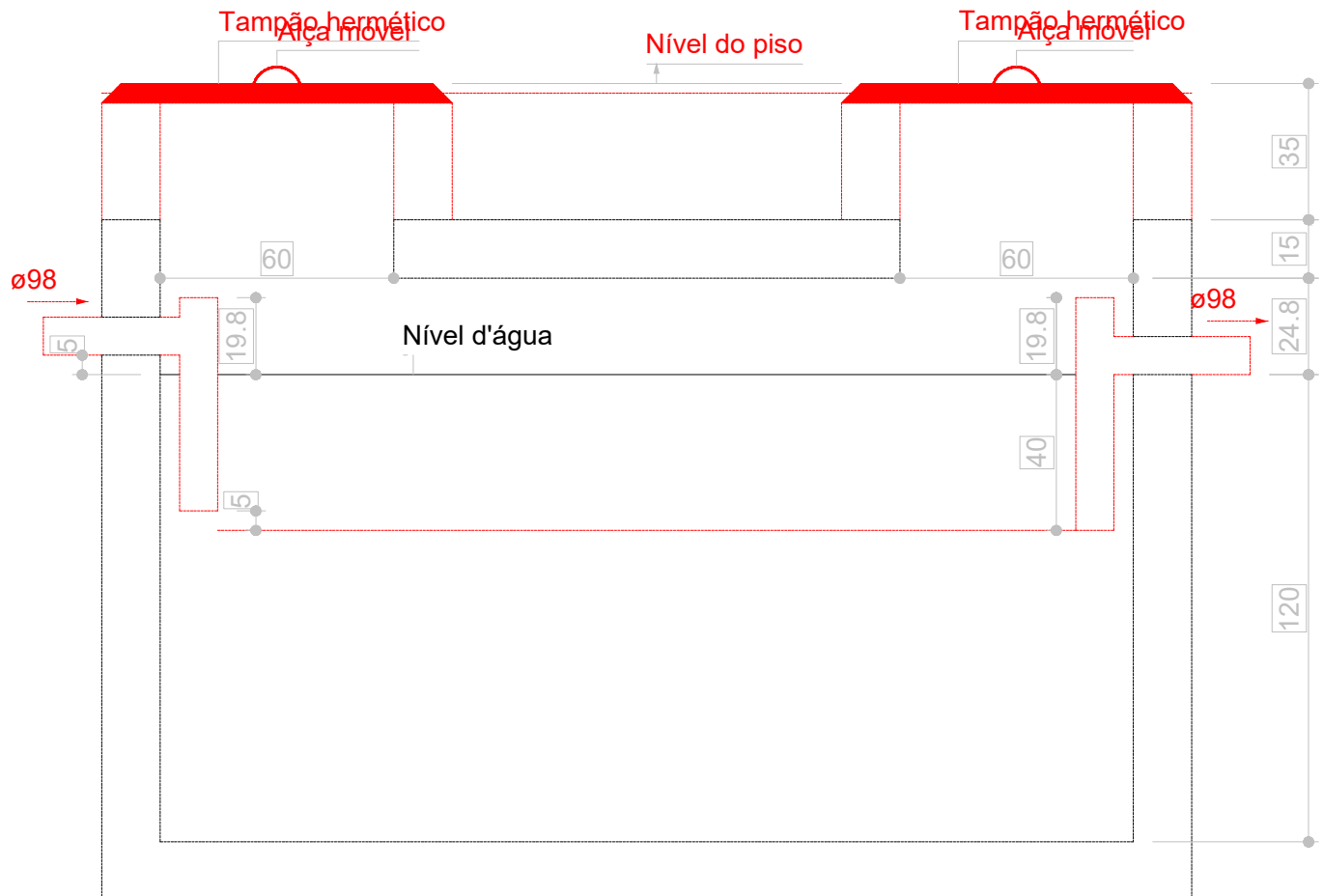
Tanque séptico - Cobertura Corte 1 - ESC. 1:25
