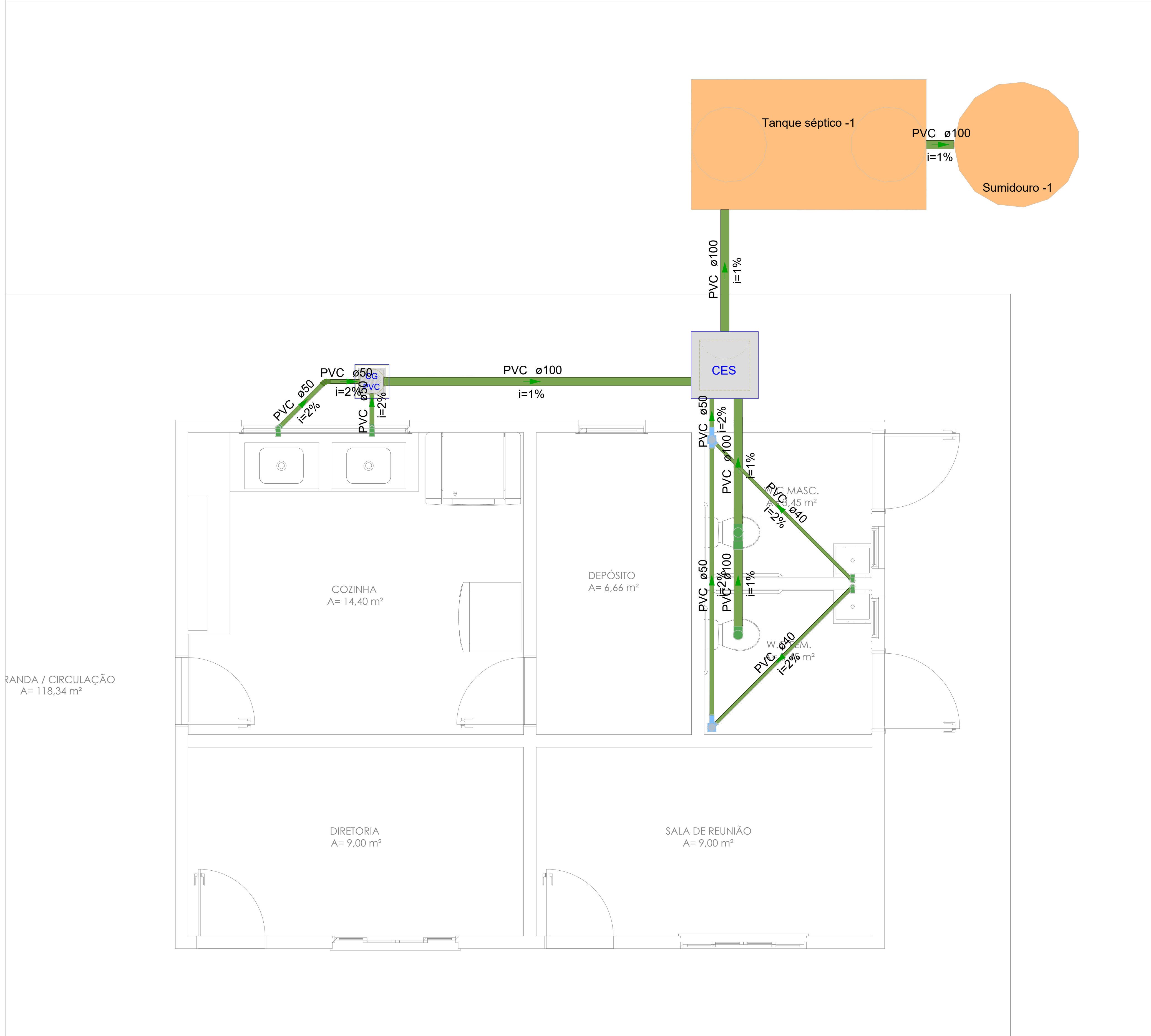
PROJETO SANITÁRIO ESC.: 1/50
