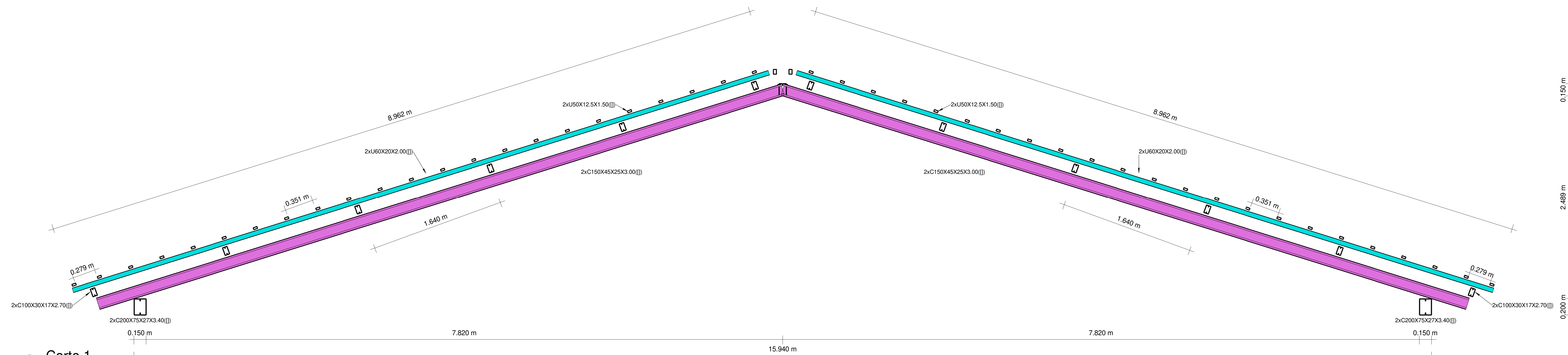
3 Corte 1 1 : 20
