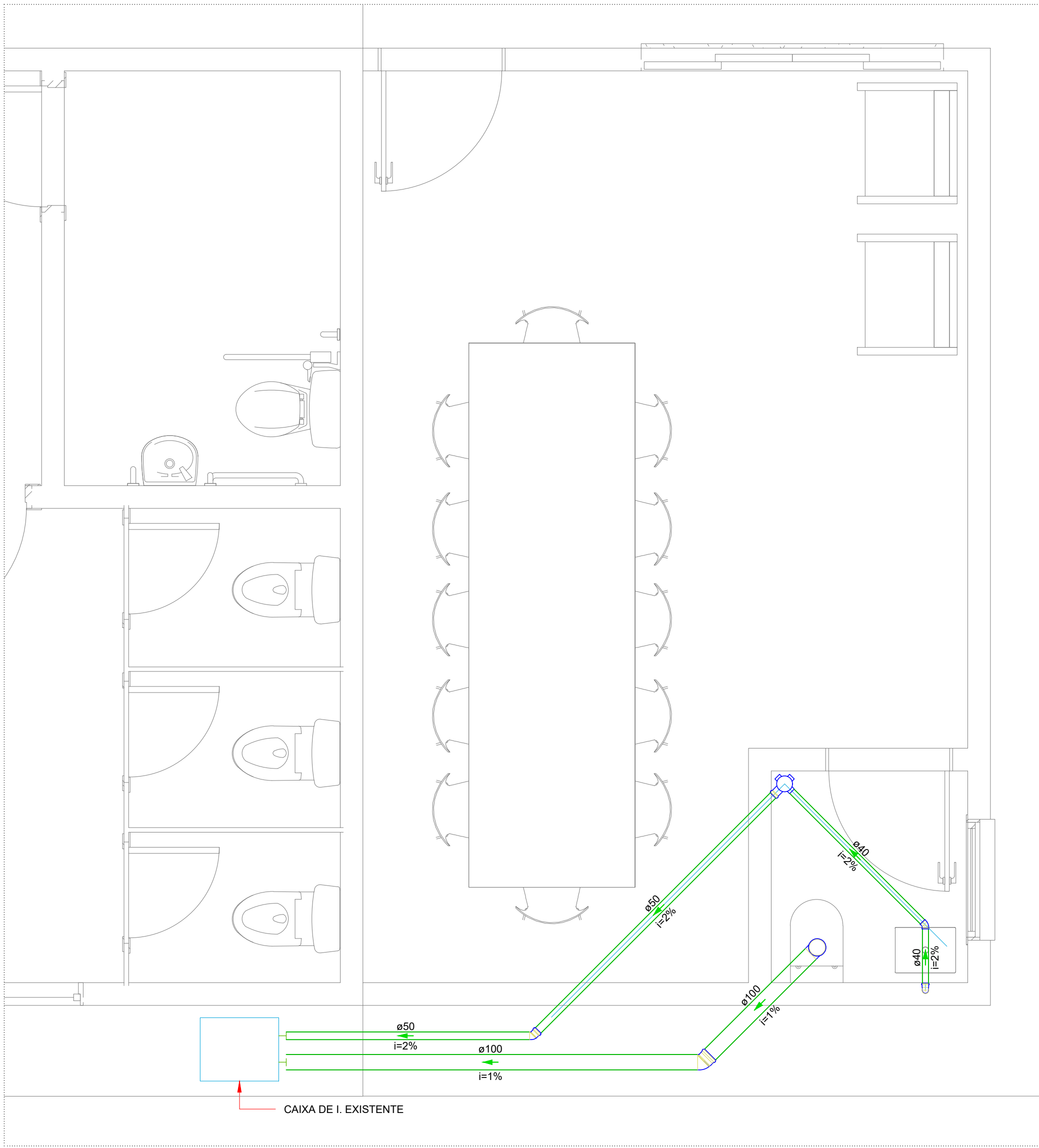
DET. SANITÁRIO 1 Escala 1:25
