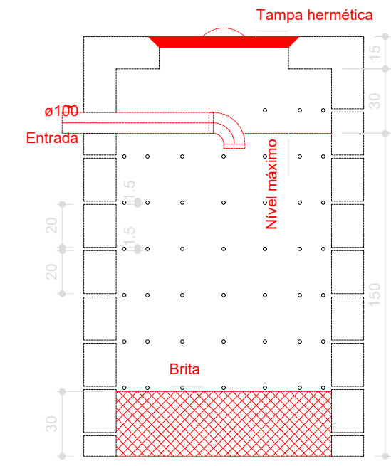
Sumidouro - FORRO Corte 1 - ESC. 1:25
