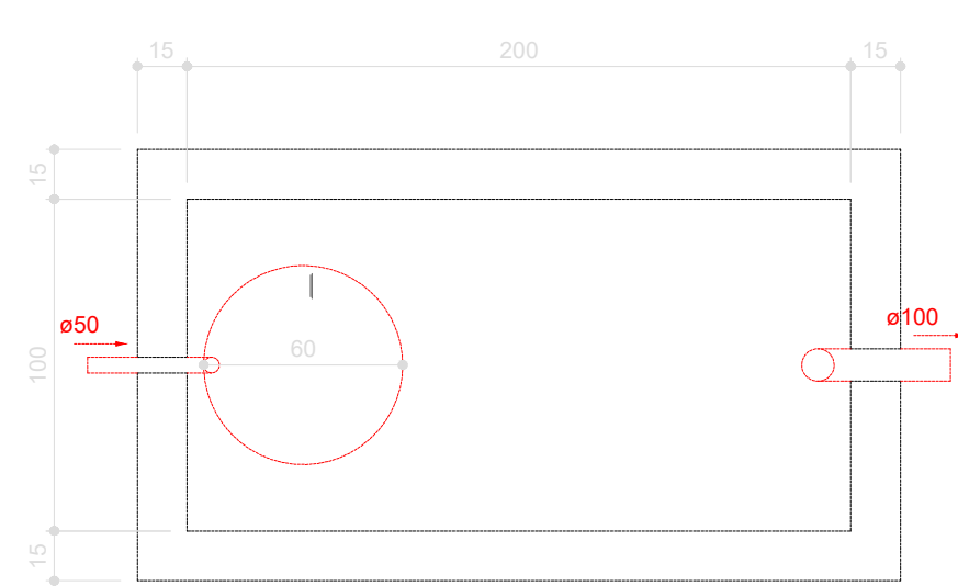
Tanque séptico - FORRO Planta baixa - ESC. 1:25
