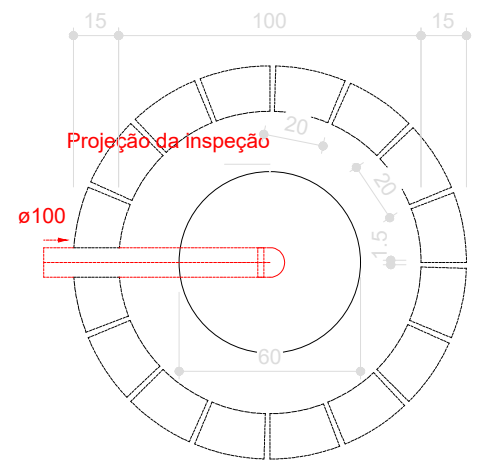
Sumidouro - FORRO Planta baixa - ESC. 1:25
