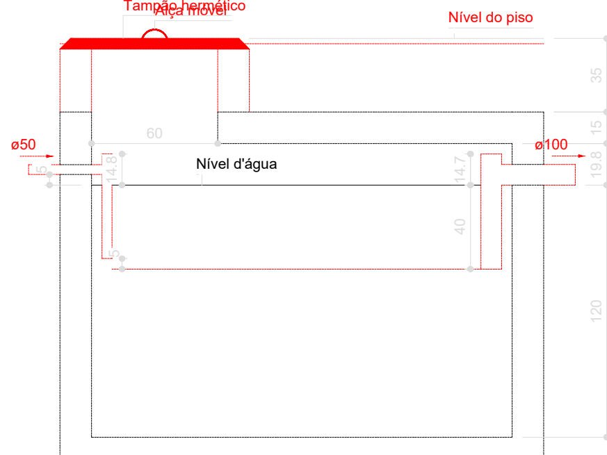
Tanque séptico - FORRO Corte 1 - ESC. 1:25
