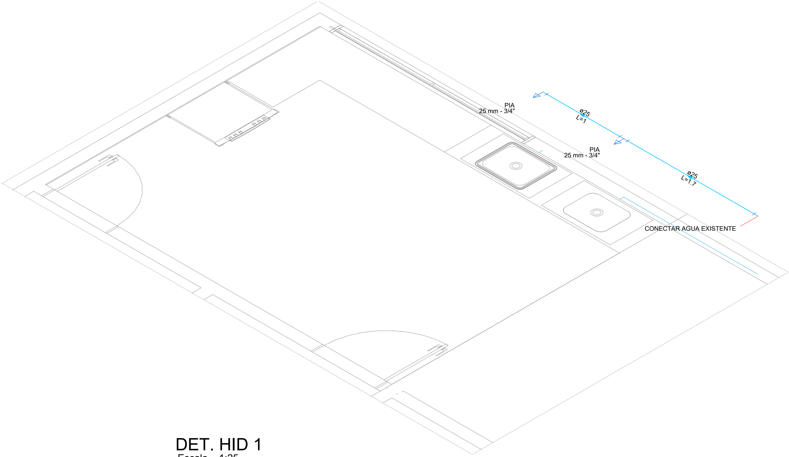
DET. HID 1
