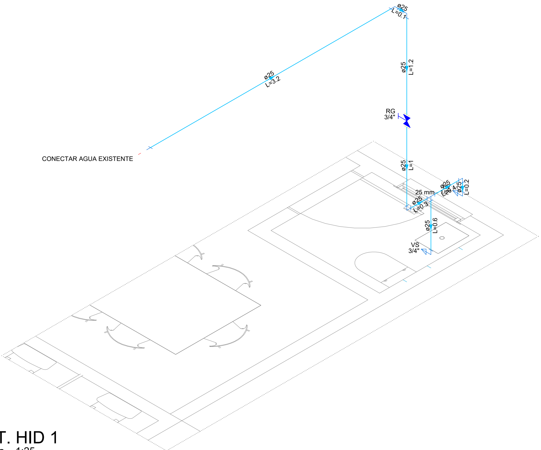
DET. HID 1
